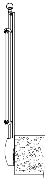
En nez de dalle.
