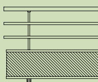
Avec double lisse intermédiaire
