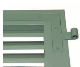
PENTURES ENTAILLÉES
